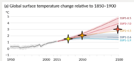
Figure 4 : Changement des températures de surface sur le globe (source GIEC 2021) selon différents scénarios climatiques. Les valeurs de niveau de réchauffement de la TRACC sont repérées par des losanges jaune, orange et rouge.
